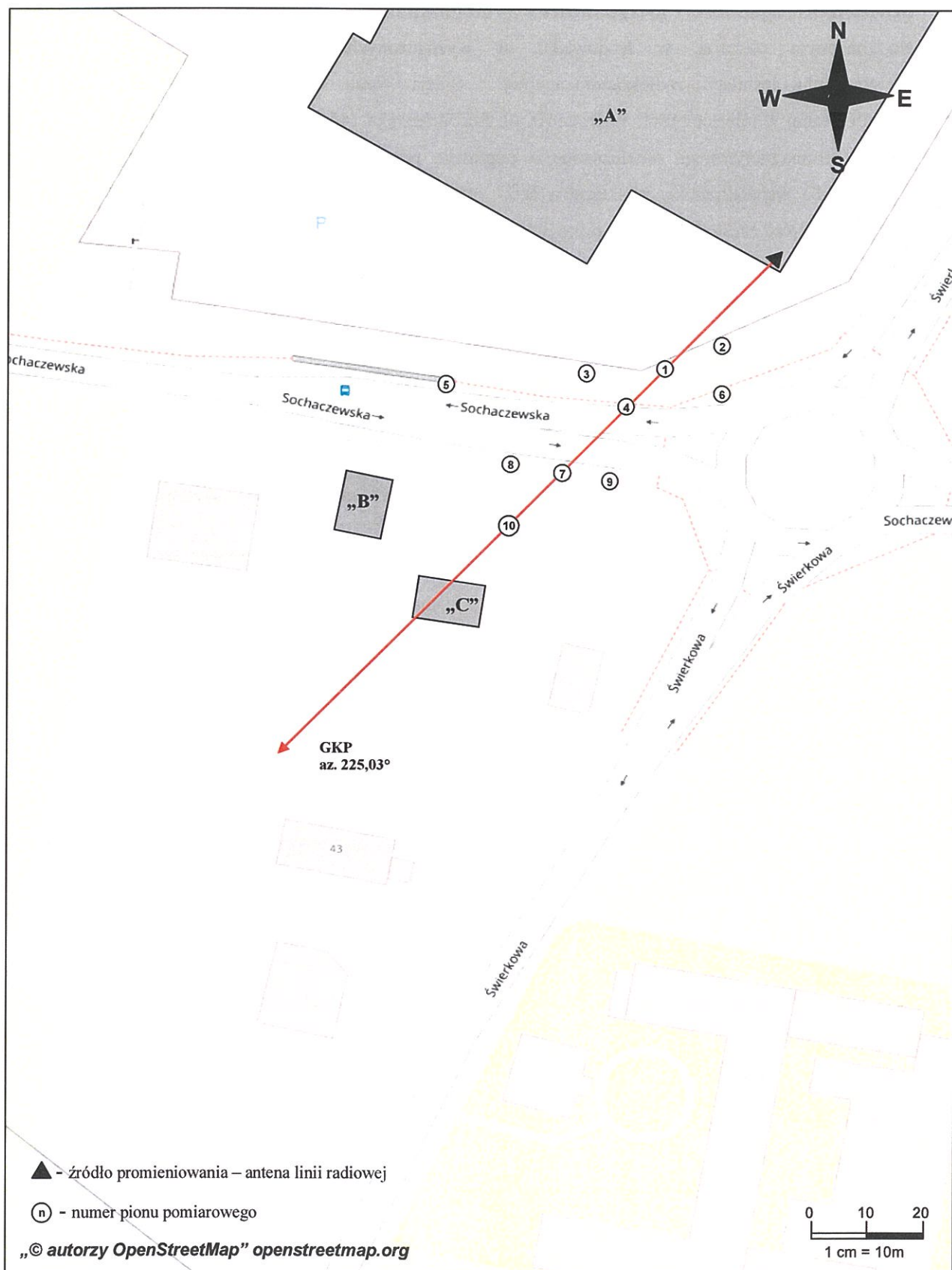
Rys. 1. Usytuowanie punktów i pionów pomiarowych w otoczeniu instalacji radiokomunikacyjnej Stacja Netia OZAIB034-OZAIM00031ANT003 Wieruchów, ul. Sochaczewska 144
